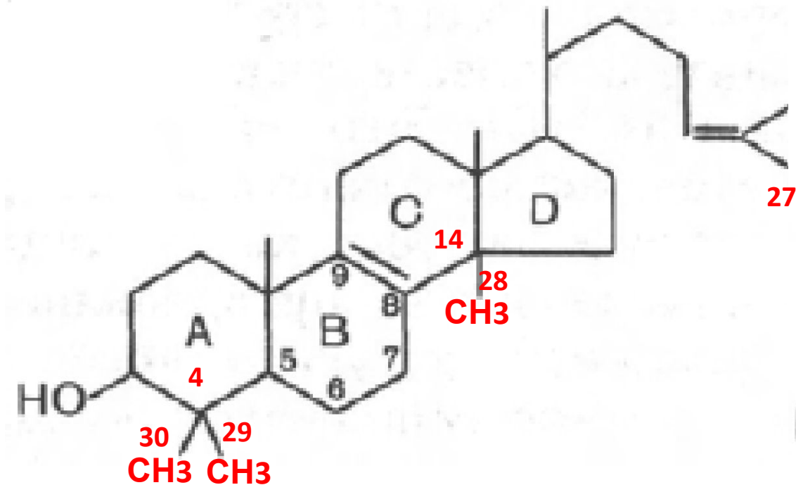
Ланостерин C30
