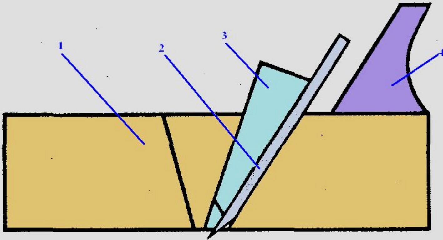
Рис.3. Устройство рубанка. 1 - колодка; 2 - нож; 3 - клин; 4 - ручка.
