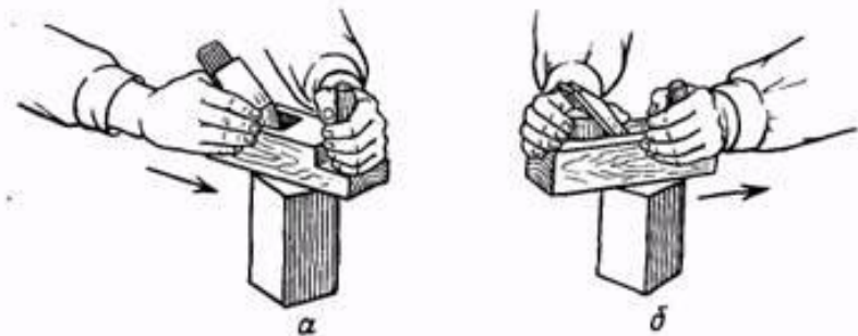
Рис. 22. Строгание торца от себя ( а ) и на себя ( б )
