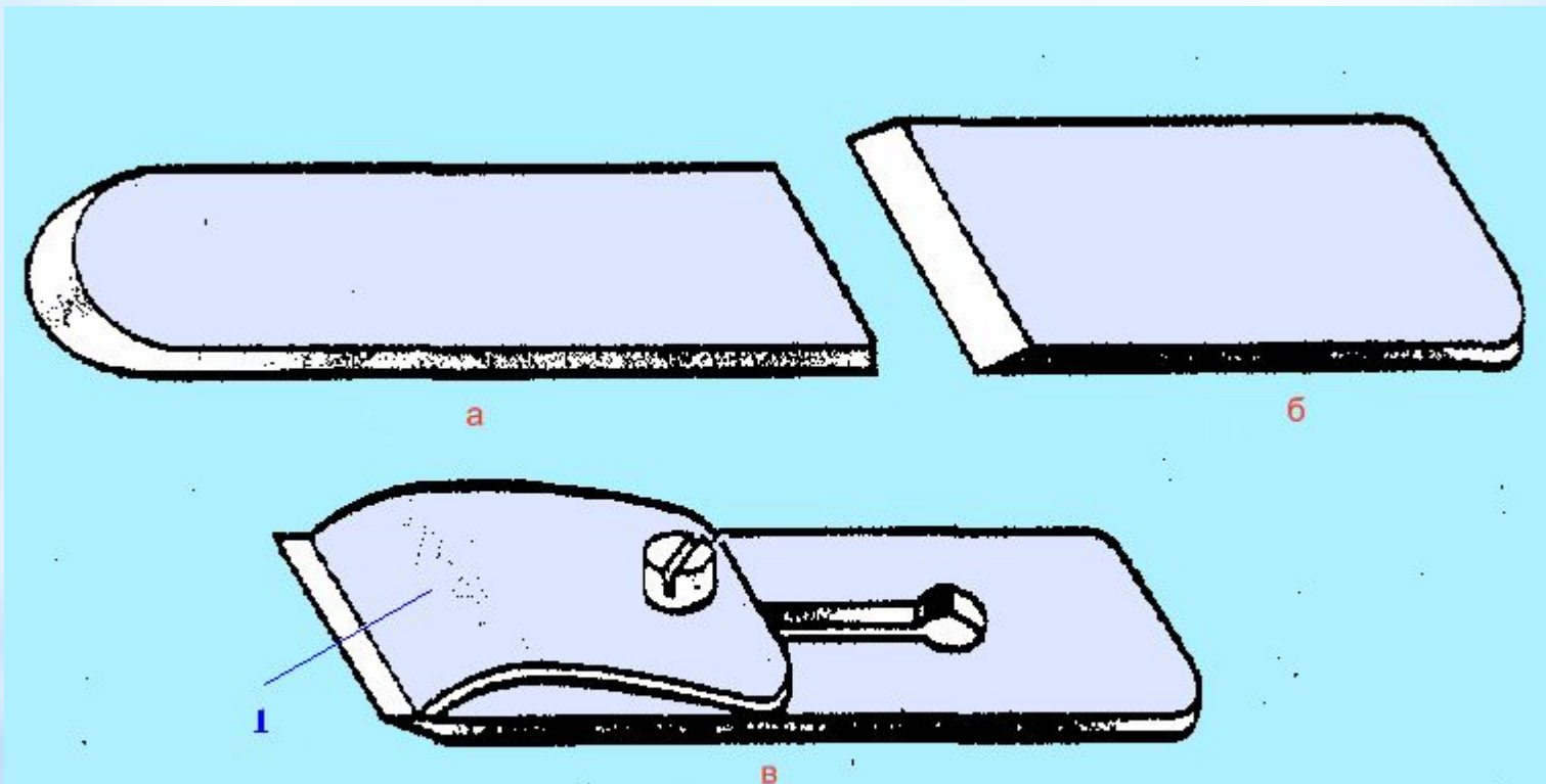
Рис.2. Ножи: а - шерхебеля; б - рубанка; в - рубанка с стружколомателем; 1 - стружколоматель.
