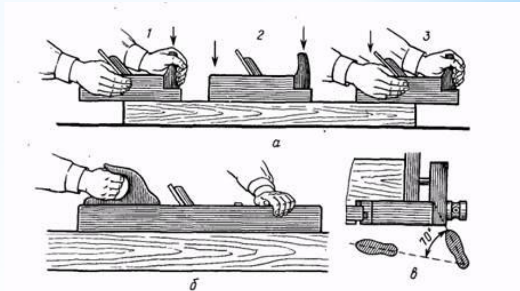
Рис. 21. Приёмы строгания:
