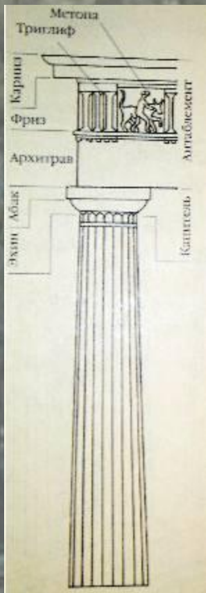
Капитель дорического ордера
