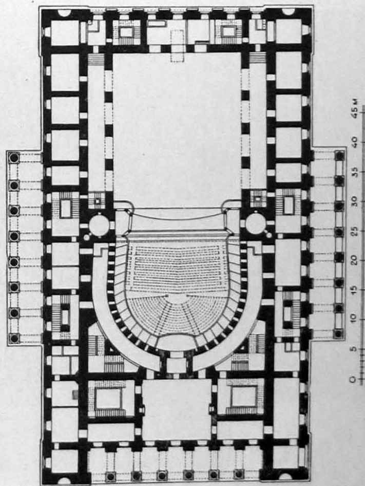
Бывш. Александринский театр в Ленинграде. План бельэтажа Арх. К. Росси
