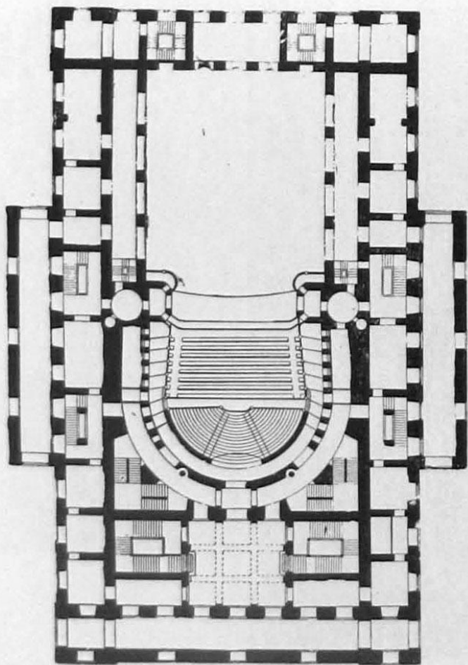
Бывш. Александринский театр в Ленинграде. План партера Арх. К. Росси
