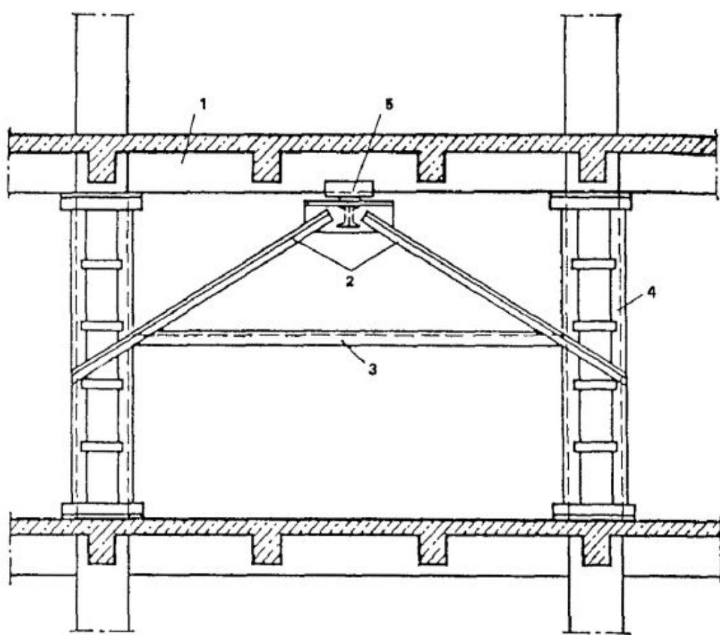
Усиление ригеля металлическими подкосами с опорой на обойму колонны
