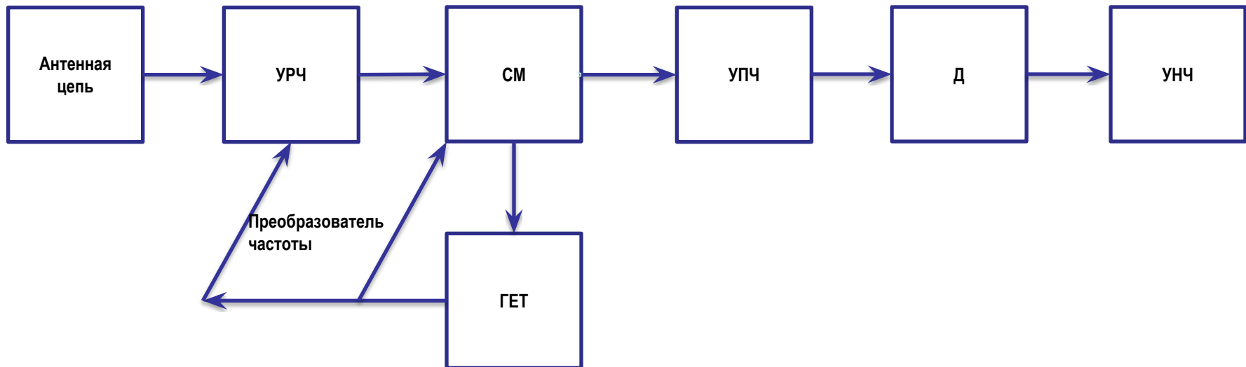
рис 1.4. Структурная схема супергетеродинного приемника.
