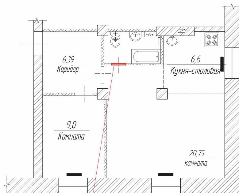
План квартиры после перепланировки
