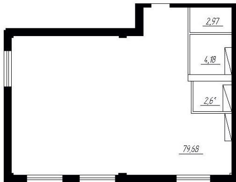
План квартиры после перепланировки (вариант 3)
