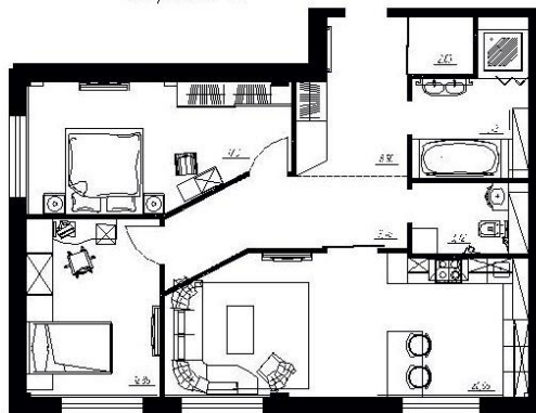
План квартиры после перепланировки (вариант 2)
