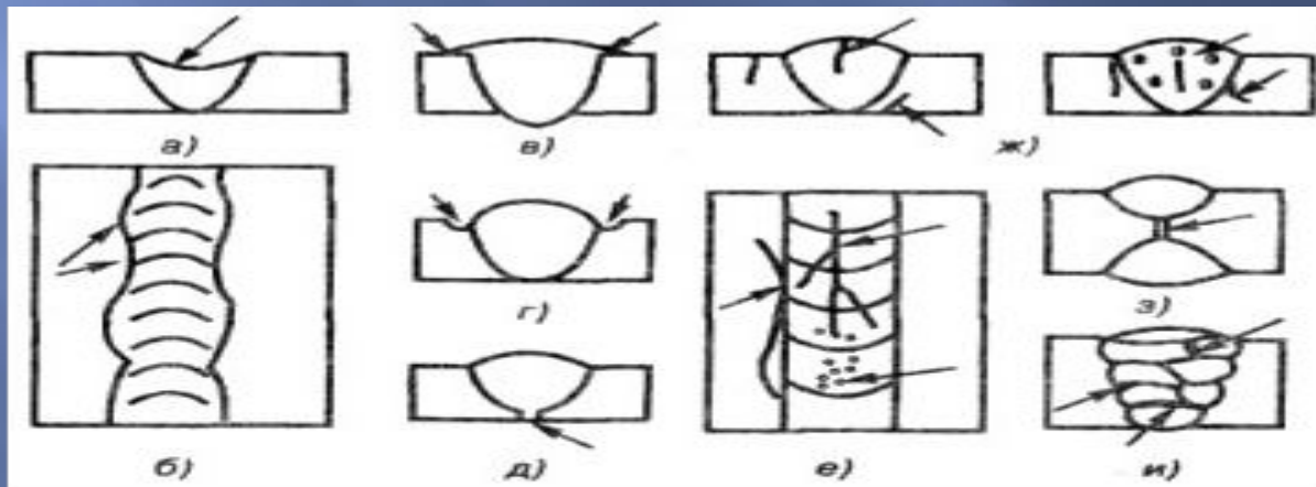
Рис. 1. Виды дефектов сварных швов: а - ослабление шва б - неравномерность ширины, в - наплав, г - подрез, с - непровар, с - трещины и поры, ж - внутренние трещины и поры, з - внутренний непровар, и - шлаковые включения
