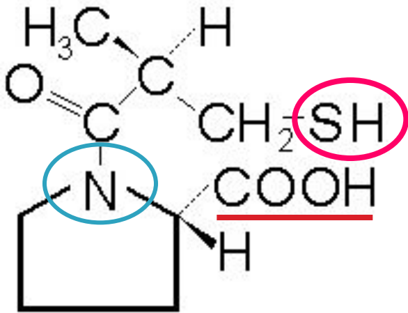
Каптоприл
