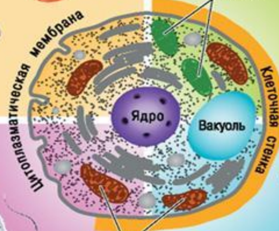
Митохондрии
