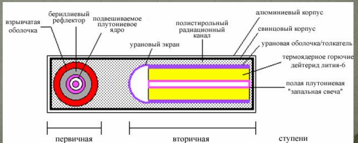
рис. 1 Двухэтапная схема радиационной имплозии Теллера-Улама
