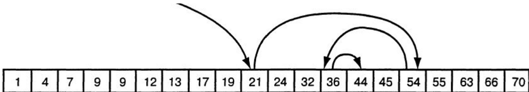
Двоичный поиск элемента со значением 44
