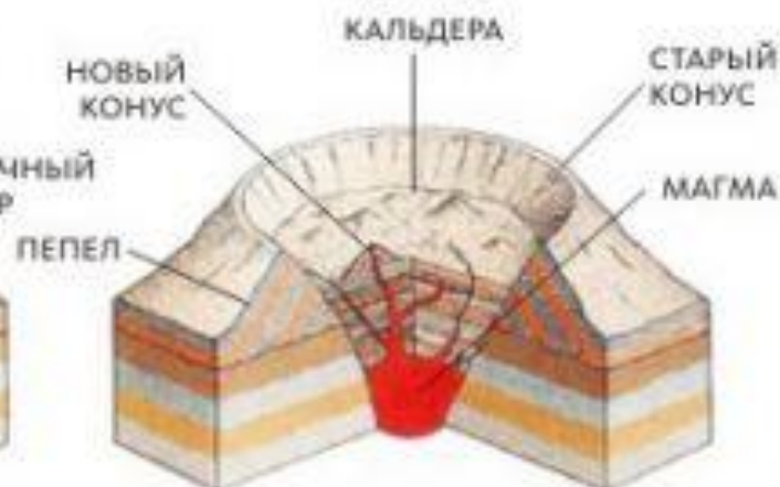
Кальдера
