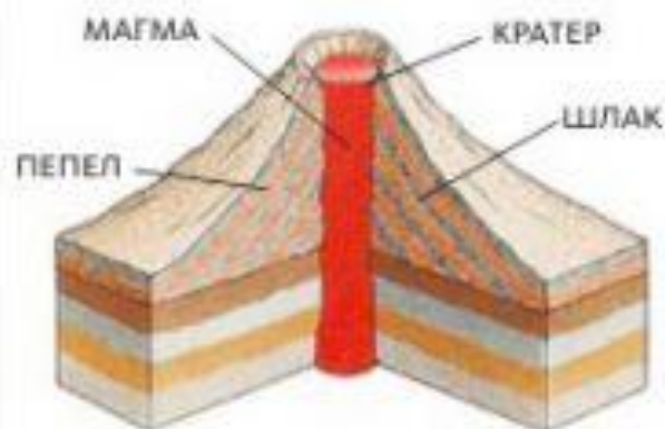
Шлаковый конус
