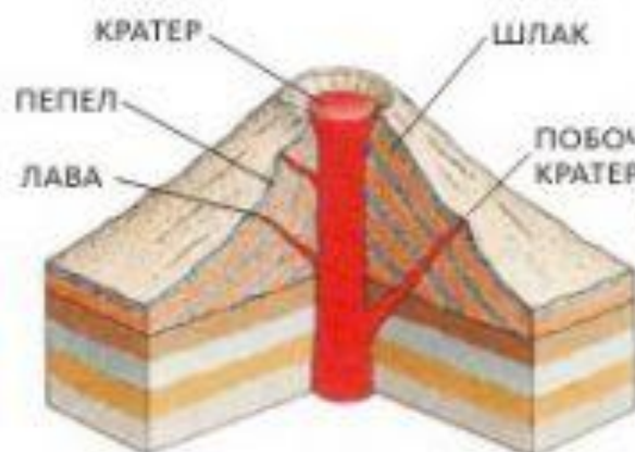
Стратовулкан
