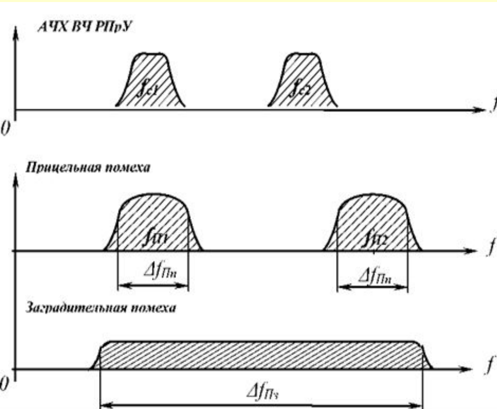
Прицельная и заградительная активные помехи
