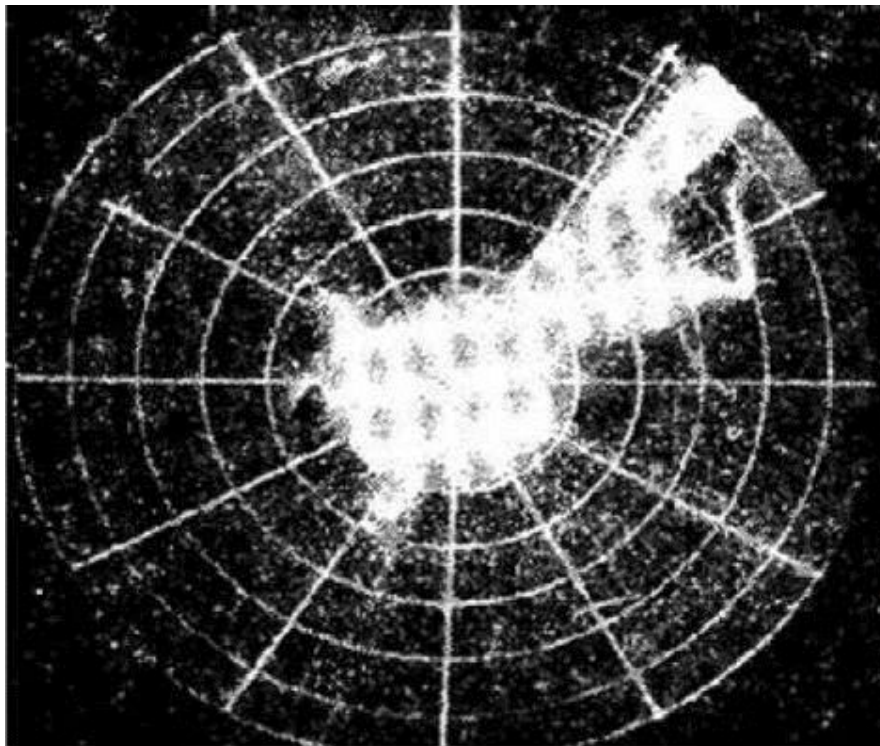
Экран ИКО при воздействии комбинированных помех
