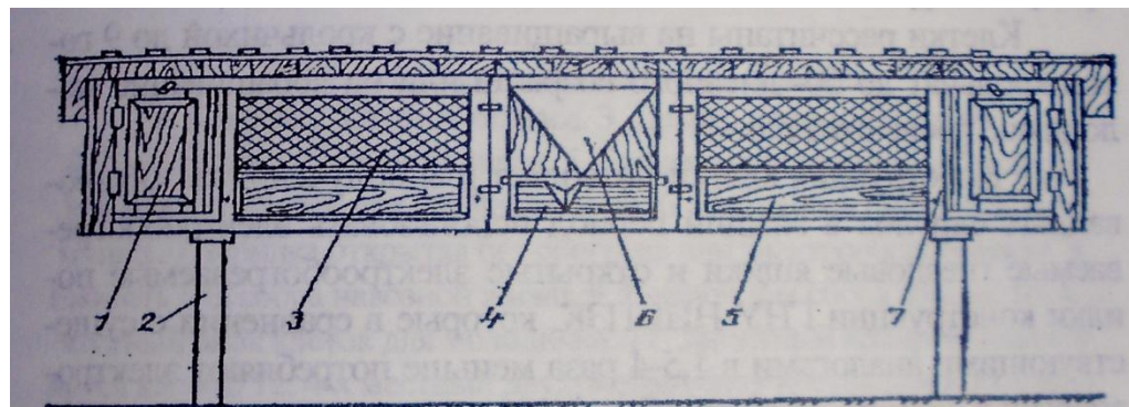
Рис. 1. Двухместная клетка для взрослых крольчих с гнездовым отделением:
