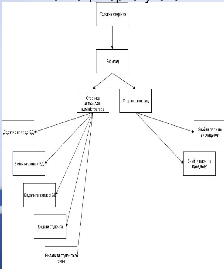
Спроектована схема навігації користувача
