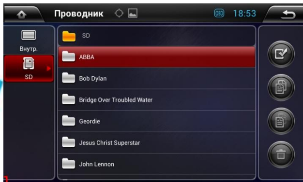
Интерфейс «Проводник»
