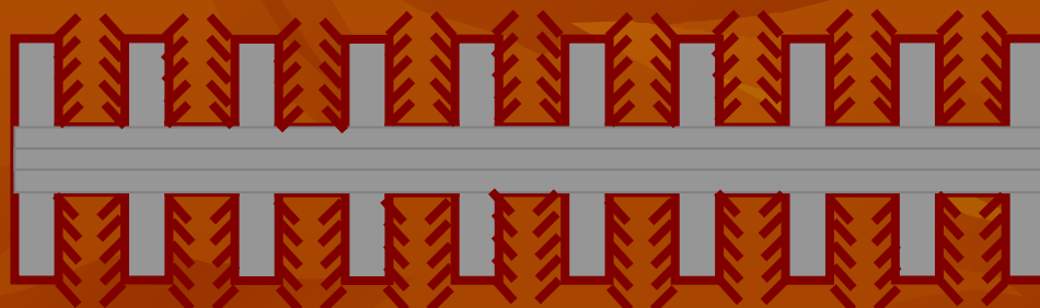
Фиг. 2. Схема электрода Планте с использованием поверхностного промежуточного полимерного слоя «ворса», как носителя активной массы. Степень развития поверхности свинца с полимерным «ворсом» - 20-30 раз.
