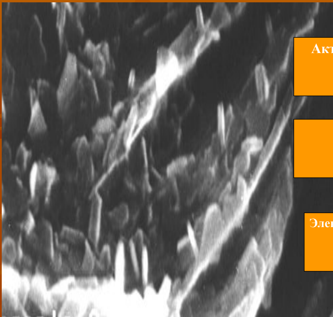
Фиг. 5. Электронная фотография активной массы (+)-электрода, на полимерном каркасе (ворс).
