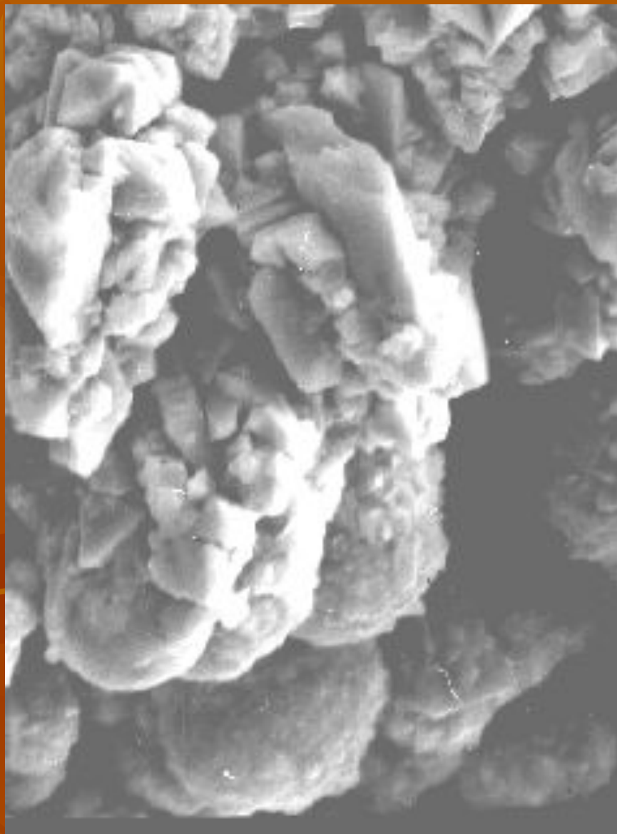
Фиг. 4. Электронная фотография типичной активной массы
