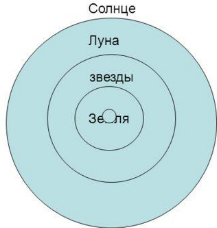
Система мира по Анаксимандру
