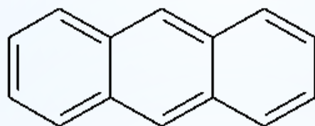
антрацен
