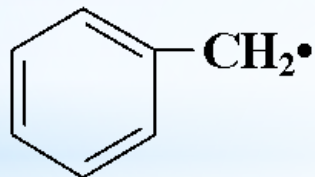
бензил
