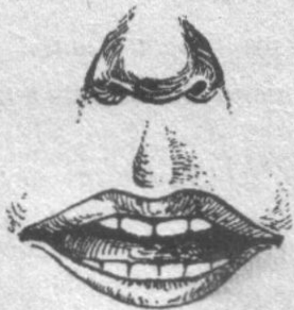
Рис. 72. Артикуляция звука и (снаружи)
