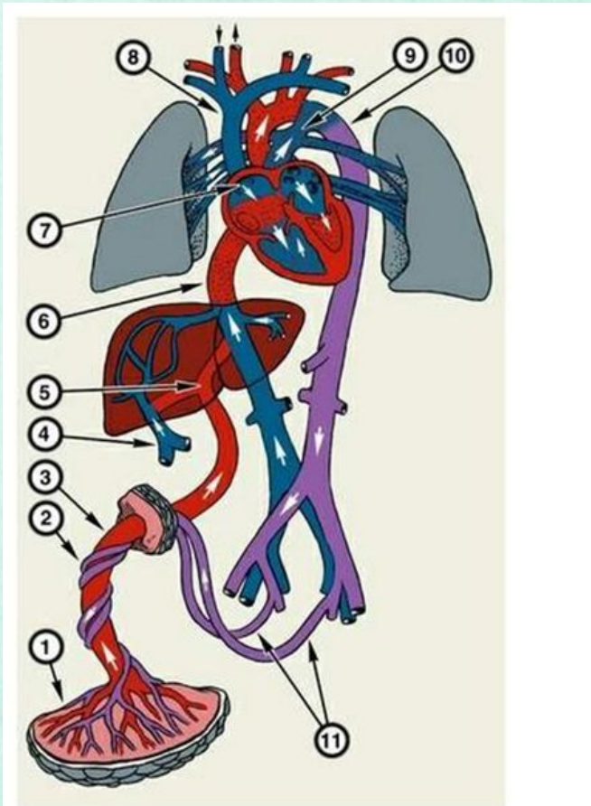
Рис. 2. Схema кровообращения плода: 1 — плацента; 2 — легочные артерии; 3 — легочная вена; 4 — воротная вена; 5 — венозный проток; 6 — нижняя полая вена; 7 — овальное отверстие; 8 — верхняя полая вена; 9 — артериальный проток; 10 — аорта; 11 — почечные артерии. Красным цветом обозначена артериальная кровь; синим — венозная; красным с синими точками — смешанная кровь, близкая по составу к артериальной; синим с красными точками и сиреневым — смешанная кровь, близкая по составу к венозной (содержание двуокиси углерода несколько меньше в крови, обозначенной сиреневым цветом).
