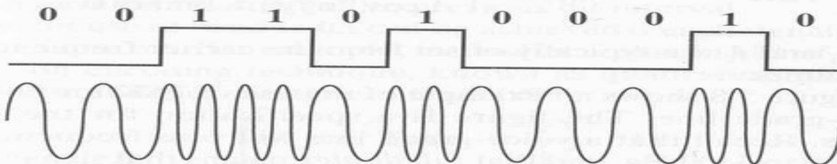
Частотная модуляция
