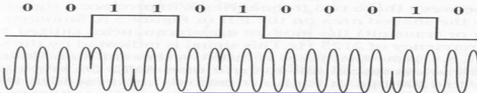
Фазовая модуляция
