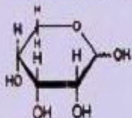
D-рибоза (Rib)
