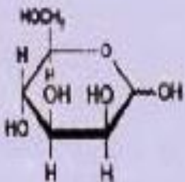
D-манноза (Man)
