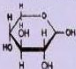
D-ксилоза (Xyl)
