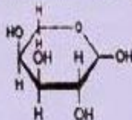
L-арабиноза (Ara)
