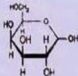
D-галактоза (Gal)
