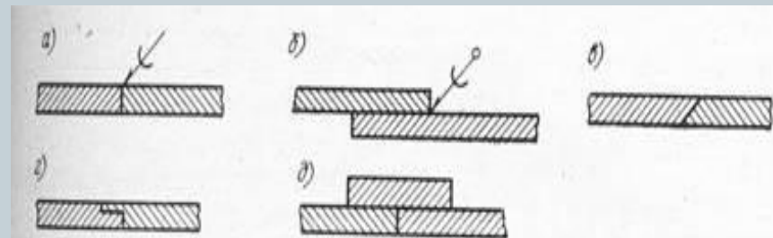
Рис. 7.4. Соединения пайкой: а — стыковое; б — внахлестку; в — «под фаску»; г — ступенчатое; д — комбинированное
