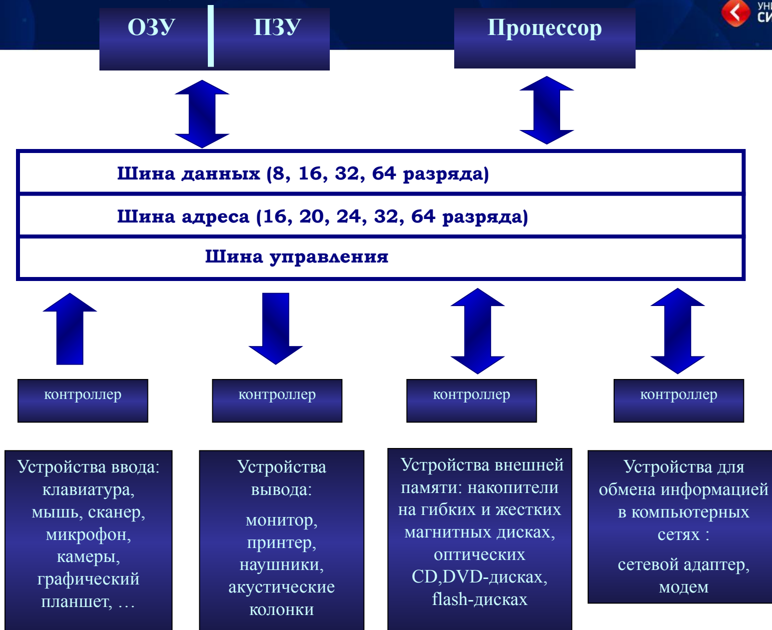
Функциональная схема компьютера, построенного по магистрально-модульному принципу
