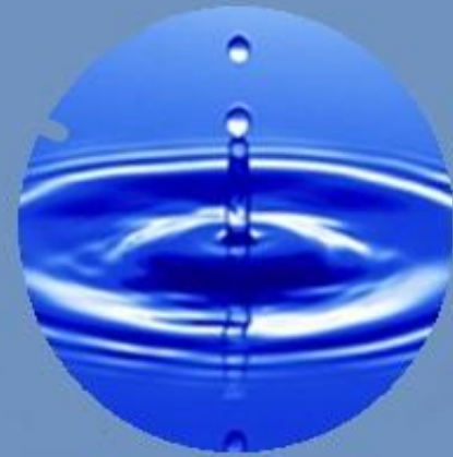
Гидросфера
