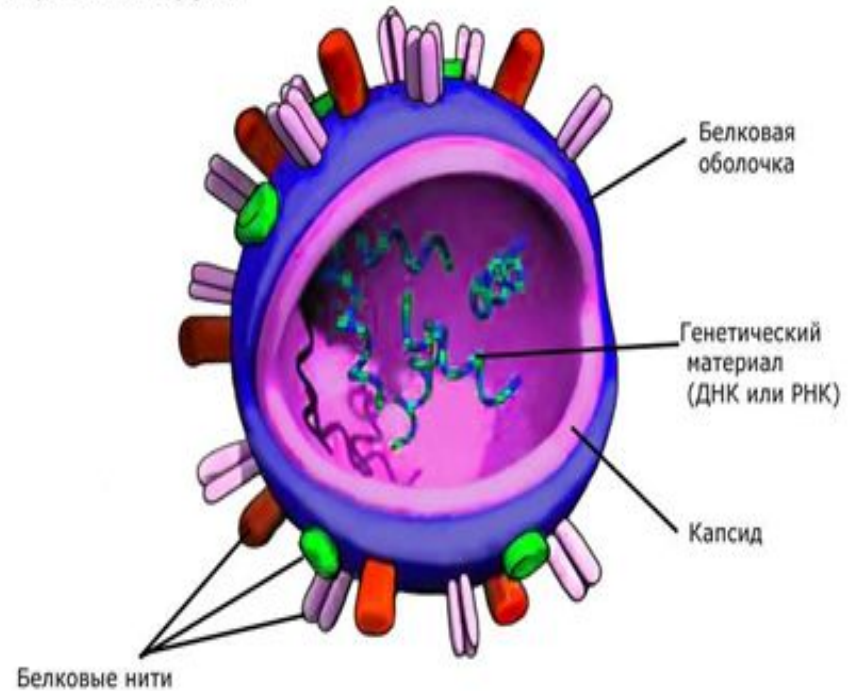
Строение вируса
