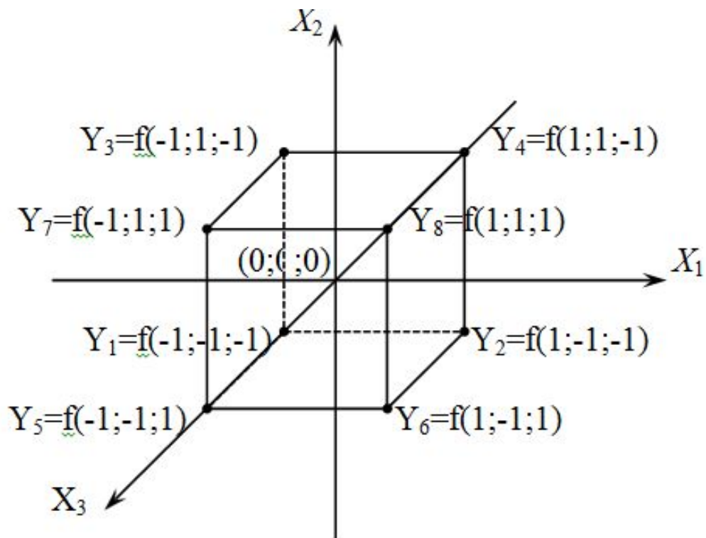
Рисунок 2 – Расположение экспериментальных точек в плане, соответствующем полиному 1-го порядка для трех независимых переменных
