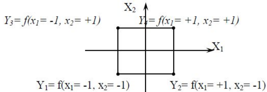
Рисунок 1 – Расположение экспериментальных точек для двух независимых факторов, варьируемых на двух уровнях
