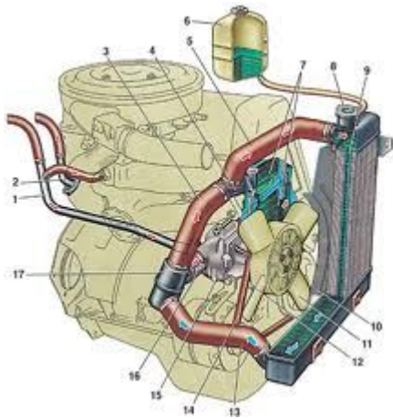
Система охлаждения автомобиля
