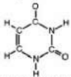
УРАЦИЛ [U]
