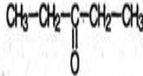
пентанон-3
