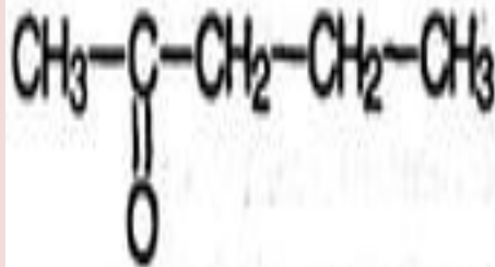
пентанон-2
