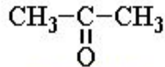
пропанон (ацетон)
