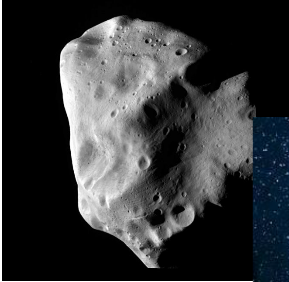
Астероид
