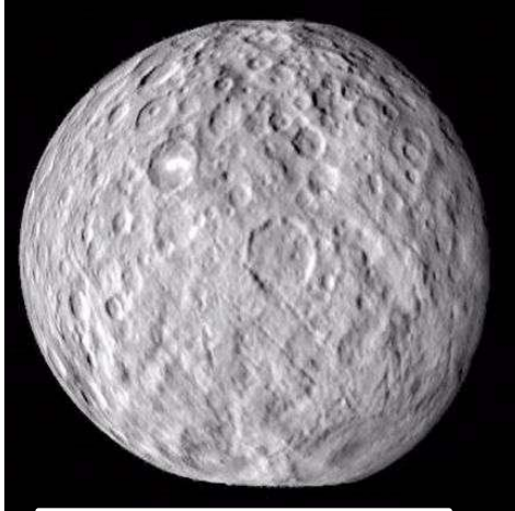
Церера
