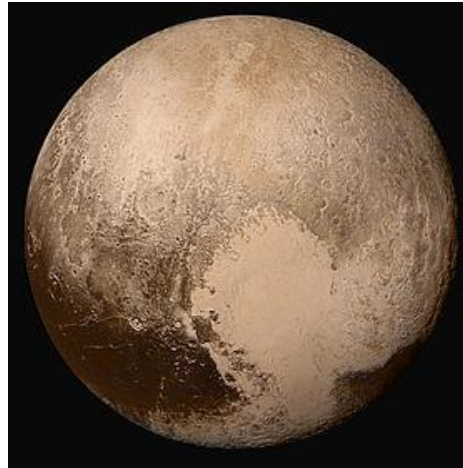
Плутон
