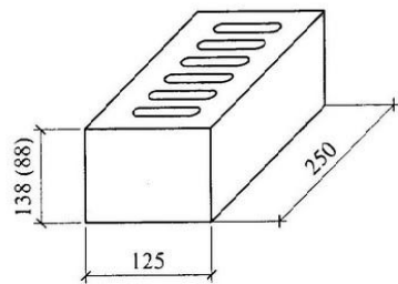
Размеры керамических пустотных камней
