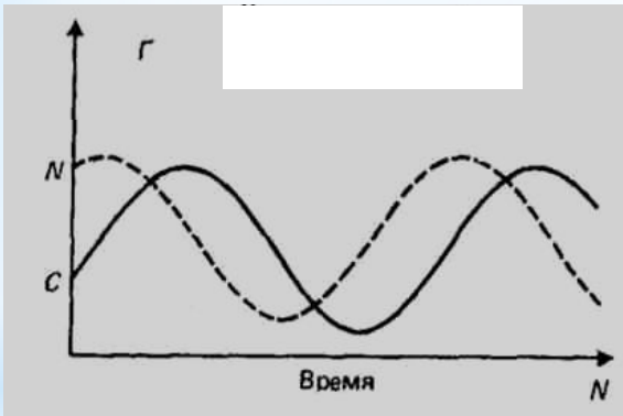
Рис. 5. Модель Лотки-Вольтерры для системы "хищник-жертва"
