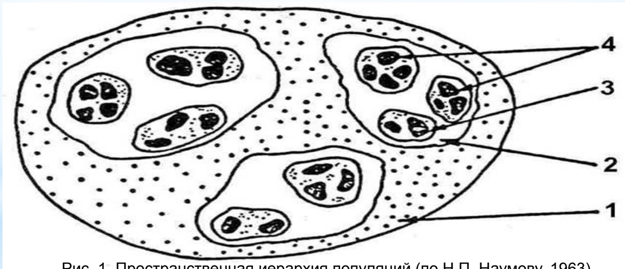
Рис. 1. Пространственная иерархия популяций (по Н.П. Наумову, 1963)
