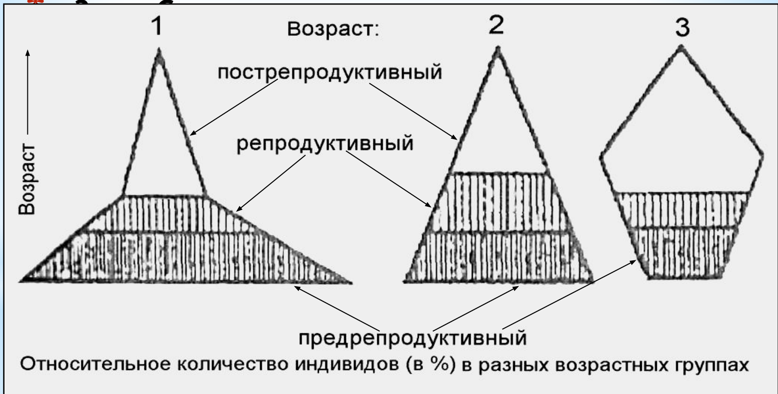
Рис. 2. Типы популяций: 1 – растущая, 2 – стабильная, 3 – сокращающаяся
