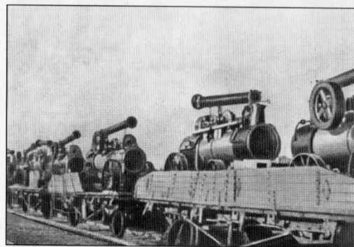
Локомотивы Людиновского завода Калужской области, изготовленные для сельского хозяйства Украины. 1945 год.
