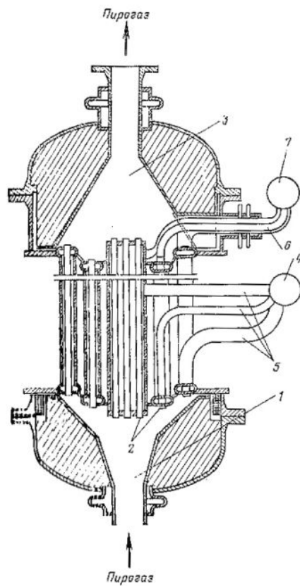
Закально-испарительный аппарат фирмы «Schmidtsche»
