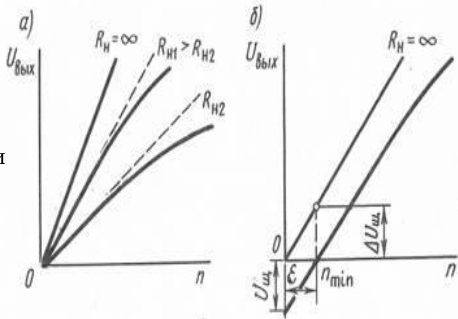
Рис. 9.6. Выходные характеристики тахогенераторов постоянного тока
