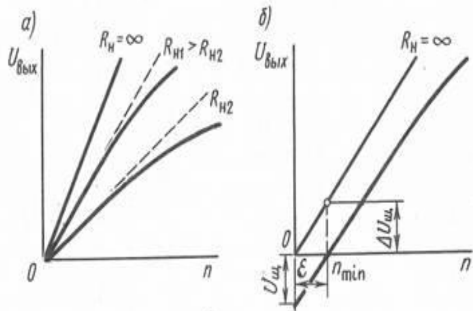
Рис. 9.6. Выходные характеристики тахогенераторов постоянного тока
