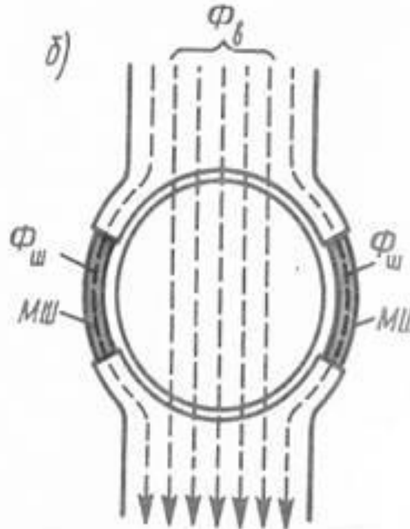
Рис. 9.7. Кривая намагничивания тахогенератора постоянного тока (а) и магнитопровод с магнитными шунтами (б)
