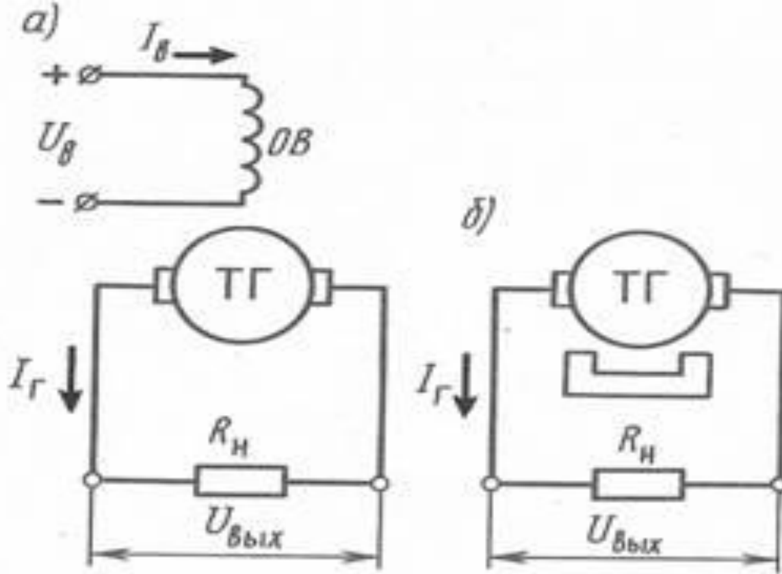
Рис. 9.5. Принципиальные схемы включения тахогенераторов постоянного тока
