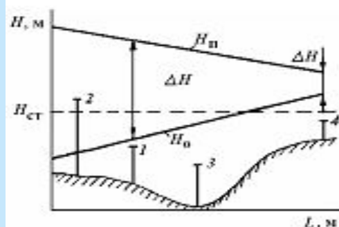
Рис. 3.4. Пьезометрический график тепловой сети: H_n , H_0 – линии напоров в подающей и обратной линиях тепловой сети в динамическом режиме; H_{ст} – линия статического режима; \Delta H – располагаемый напор на вводе одного из потребителей; 1- 4 – потребители; L – протяженность сети
