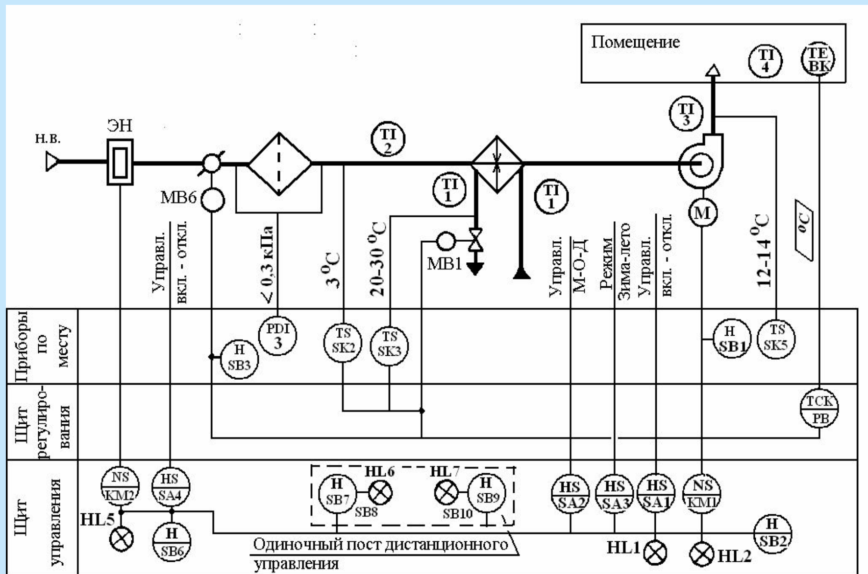
Рис. 5.1. Схема автоматизации прямоточной вентиляционной камеры
