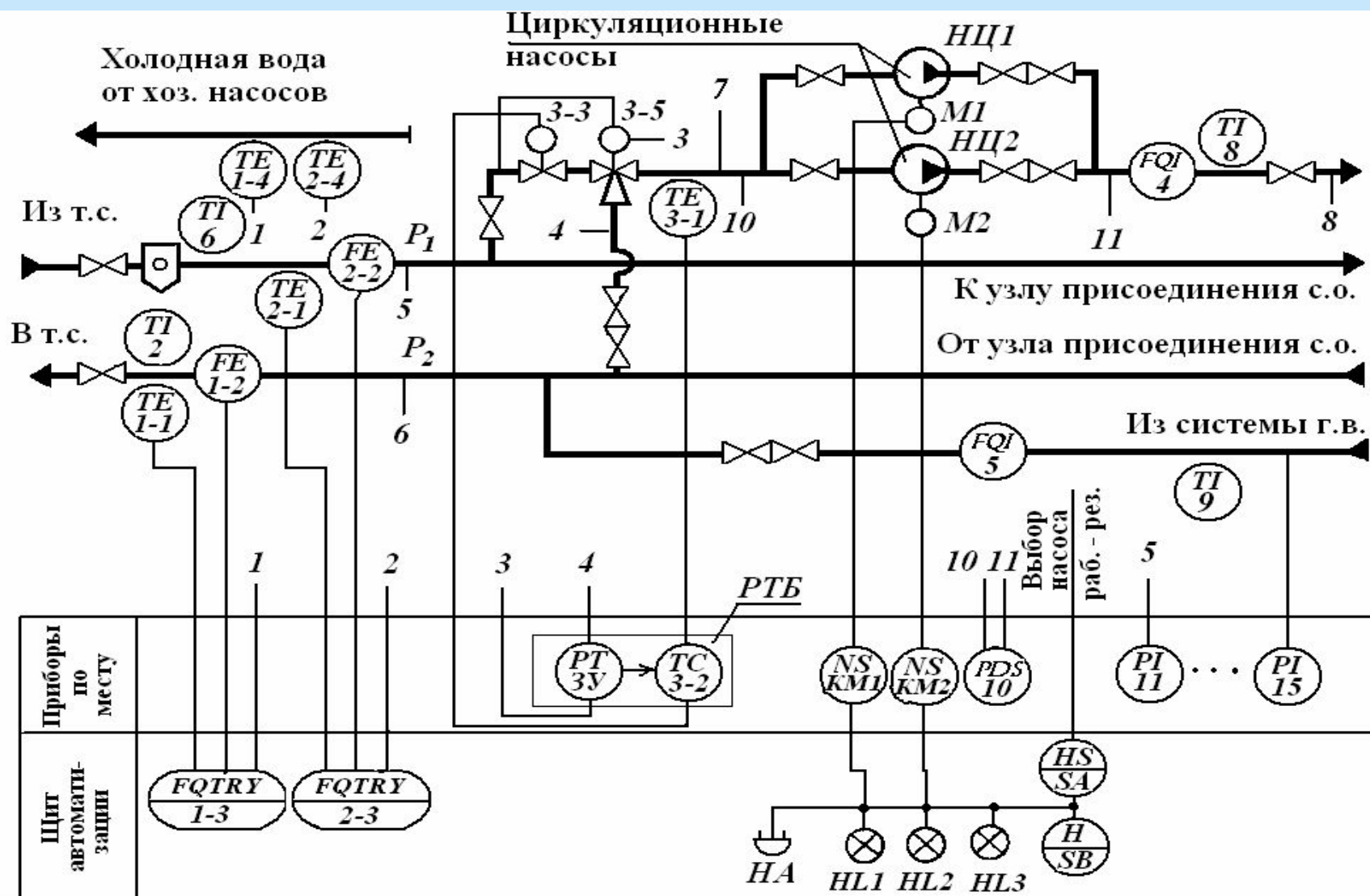
Рис. 3.3. Схема автоматизации узла присоединения системы горячего водоснабжения с непосредственным водоразбором
