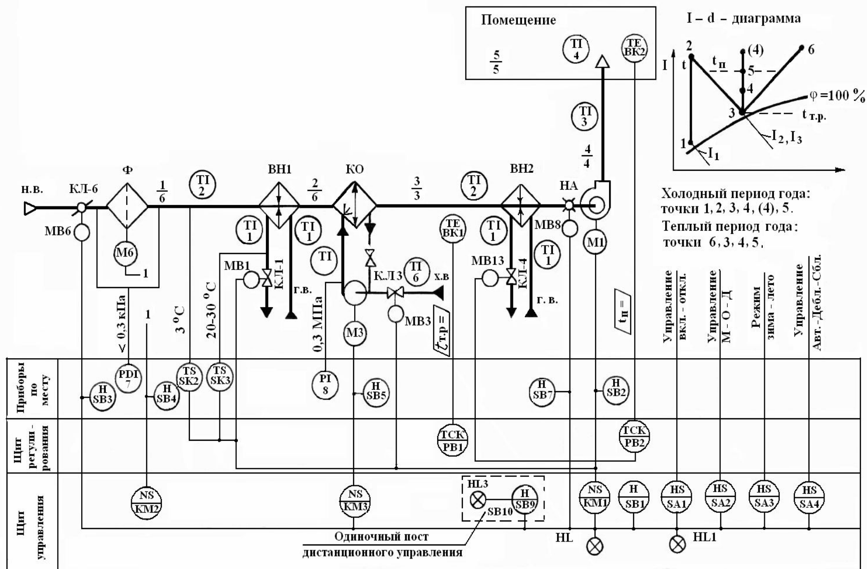
Рис. 6.1. Схема автоматизации проточного кондиционер с одной секцией воздухонагревателя первого подогрева и воздухонагревателя второго подогрева
