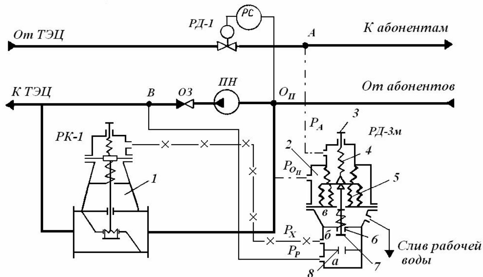
Рис. 2.7. Схема двухимпульсного регулятора подпитки системы ОРГРЭС: 1 – регулирующий клапан РК-1; 2 – регулятор давления РД-3м; 3 – регулировочный винт; 4 – пружина; 5 – сифон; 6 – сопло; 7 – заслонка; 8 – дроссель постоянного сечения
