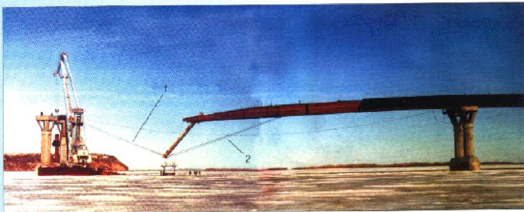
Рис. 2. Схема шпренгельного устройства, применяемого при надвигке пролетного строения:
