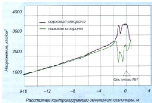
г) Напряжения в стенках балок
