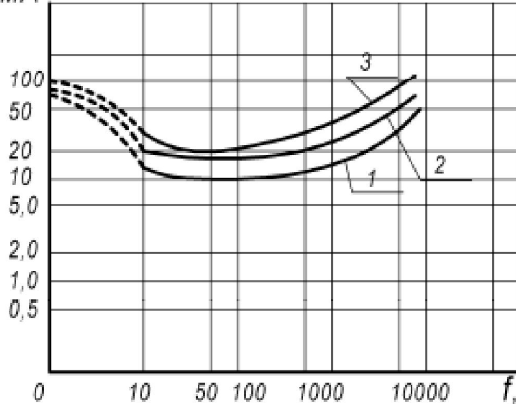
Граничные токи отпускания согласно IEC 479:
