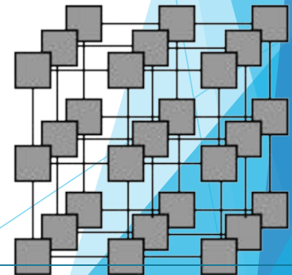
Трехмерная решетка
