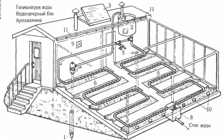
Система капельного и общего полива в солнечном вегетарии
