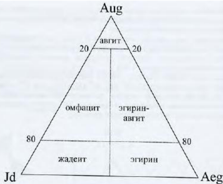
Рис. 1.50. Классификационная диаграмма щелочных клинопироксенов (Marimoto et al., 1998).
