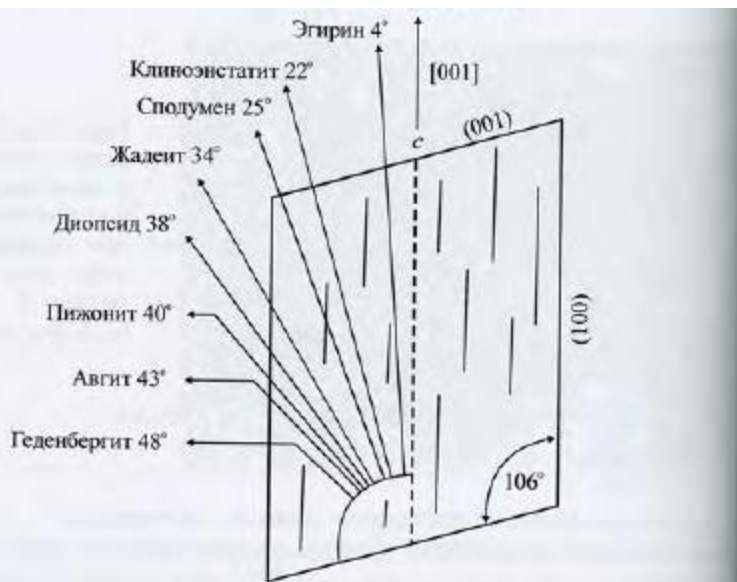
Рис. 1.52. Углы погасания пироксенов.
