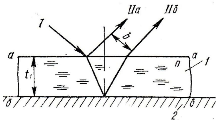
Рис. 1. Схема метода светового сечения при измерении прозрачных покрытий (или неровностей поверхности). I - ось падающего светового пучка, прошедшего щелевую диафрагму и оптическую систему; II - световые пучки, отраженные от поверхности покрытия I и основания 2.
