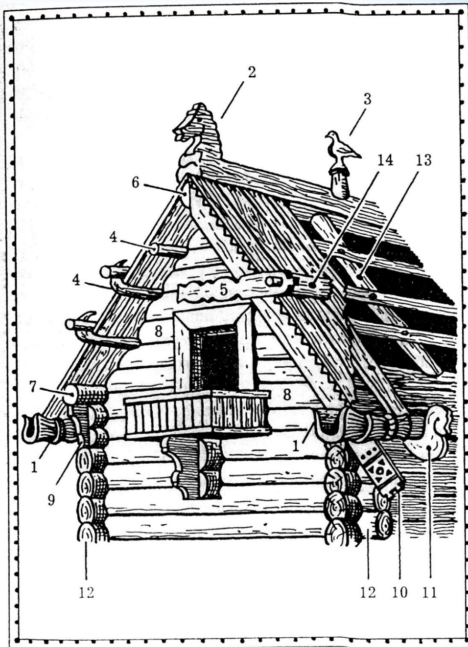
Схема устройства кровли (по М. В. Красовскому):
