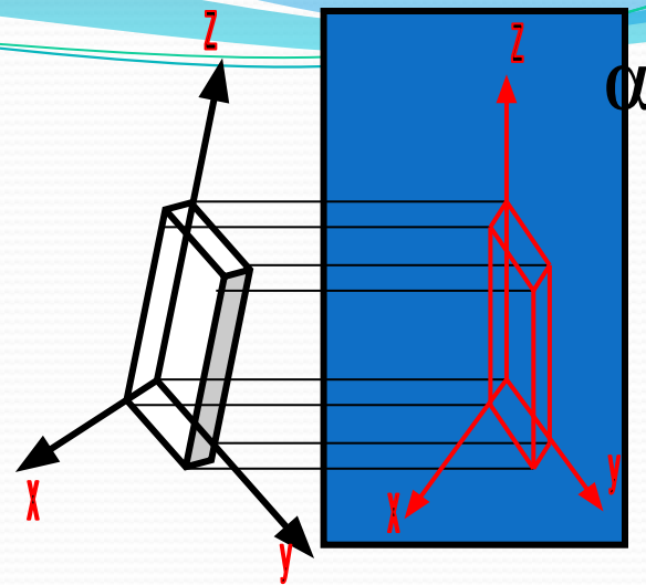
Аксонметрическая проекция
