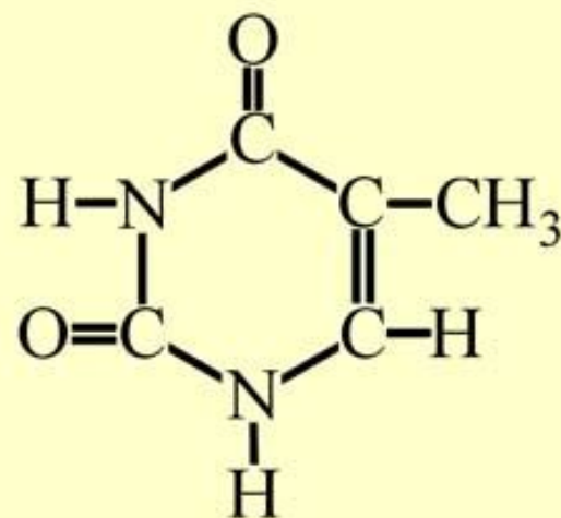
тимин
