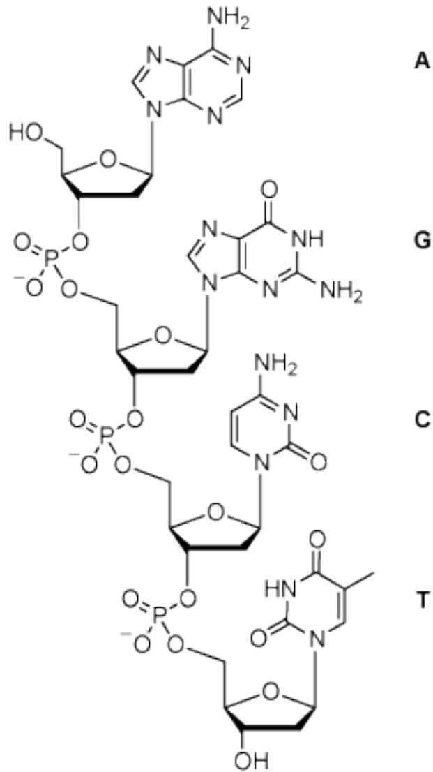
dAGCT (DNA)
