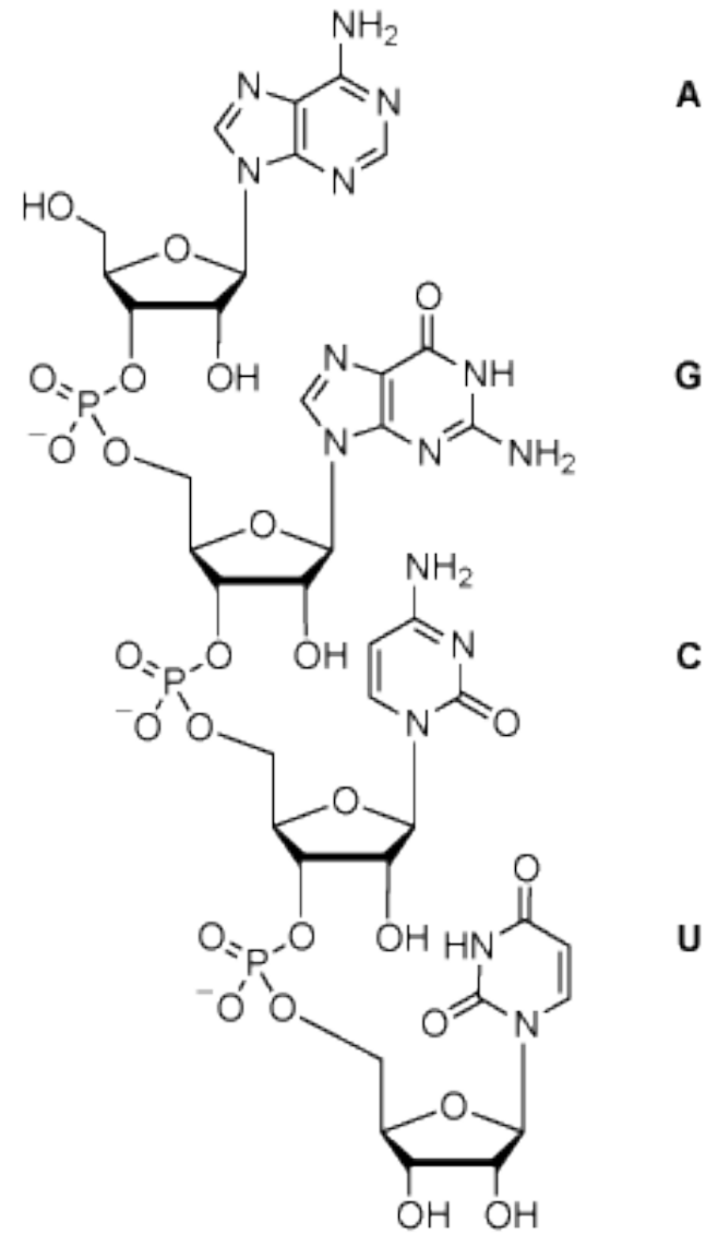
AGCU (RNA)
