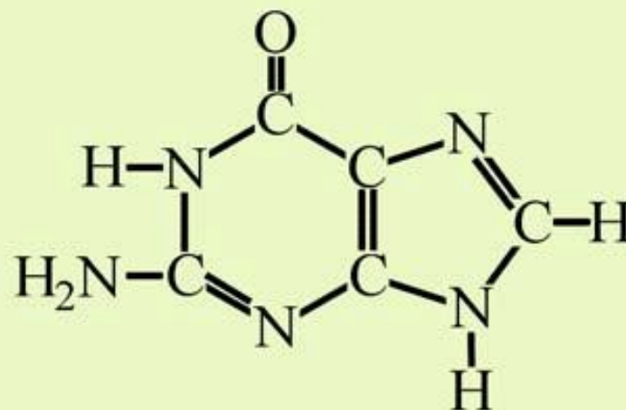
гуанин
