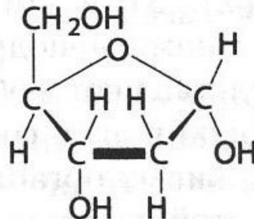
Дезоксирибоза
