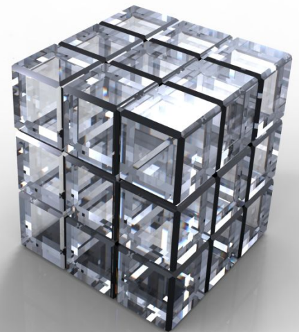
Куб
