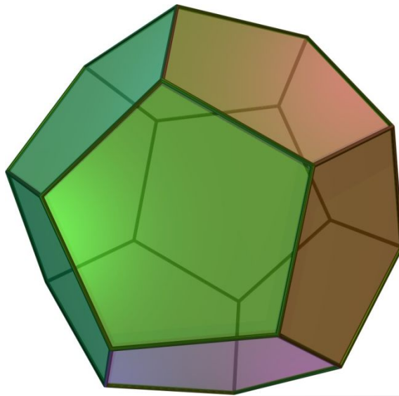
Додекаэдр
