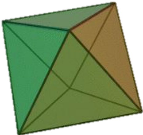
Октаэдр
