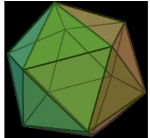
Икосаэдр
