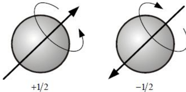
Схематическое изображение электронов с различными спинами
